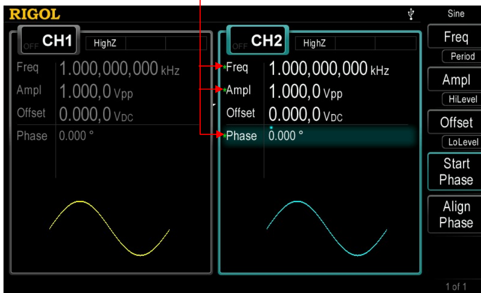
Bild 10-4 Kanalkopplung
