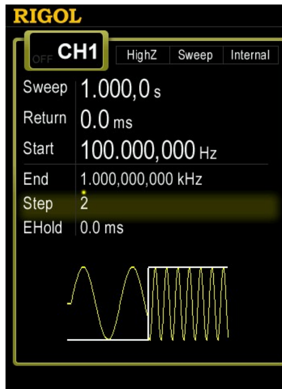
Bild 6-3 Sprung Wobbelsignal
