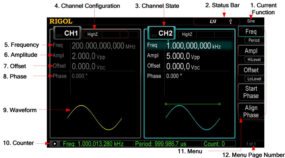
Bild 1-9 Benutzeroberfläche
