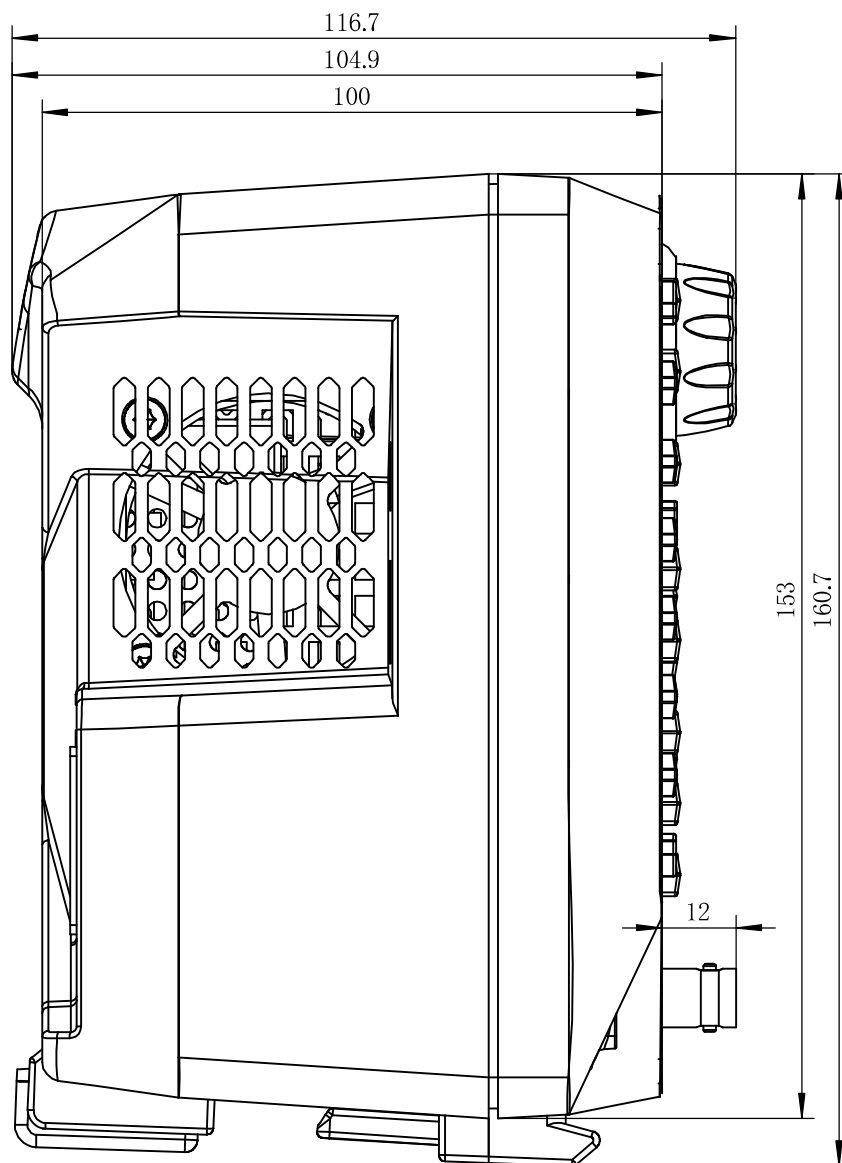
Bild 1-4 Seitenansicht
