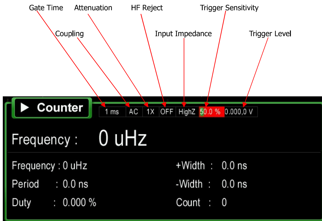
Bild 8-1 Menü Zählereinstellungen
