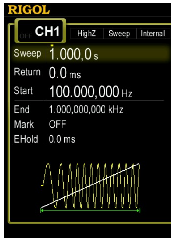
Bild 6-1 Lineares Wobbelsignal
