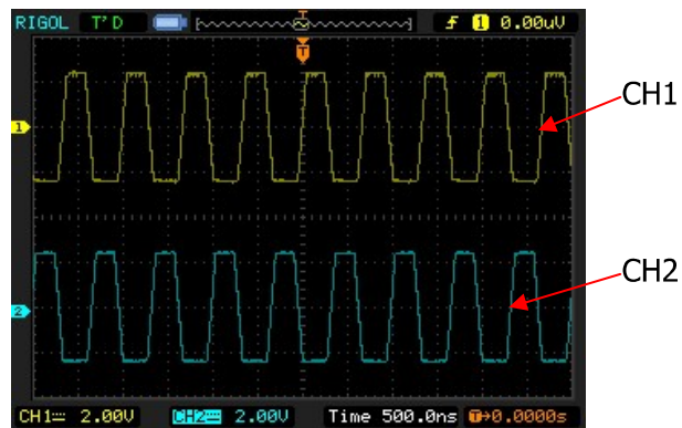
Bild 2-3 Vor Rücksetzen
