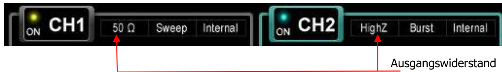
Bild 10-2 Widerstandseinstellungen
