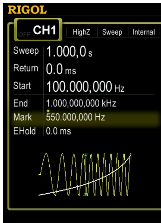
Bild 6-4 Marker Frequenz
