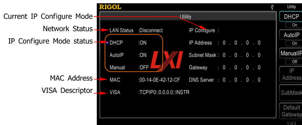
Bild 10-3 LAN Bedienoberfläche
