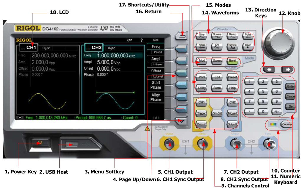
Bild 1-5 DG4000 Bedienfeld
