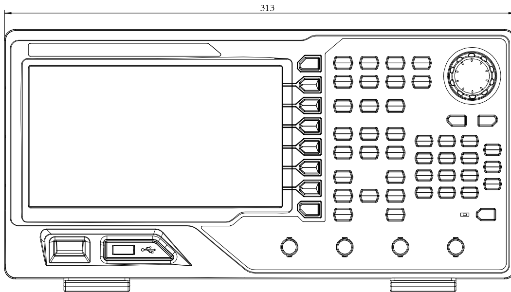
Bild 1-3 Frontansicht
