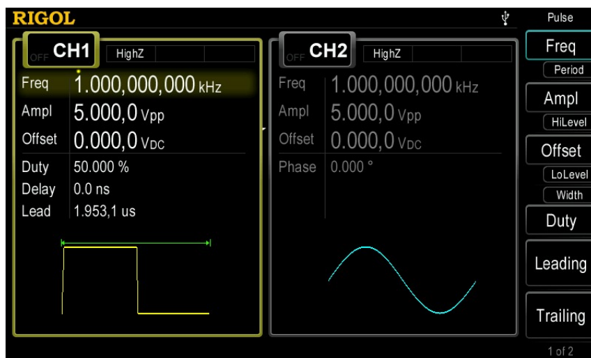
Bild 2-5 Parametereinstellung Signalform
