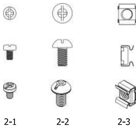
Bild 1-12 Teile Gestelleinbausatz
